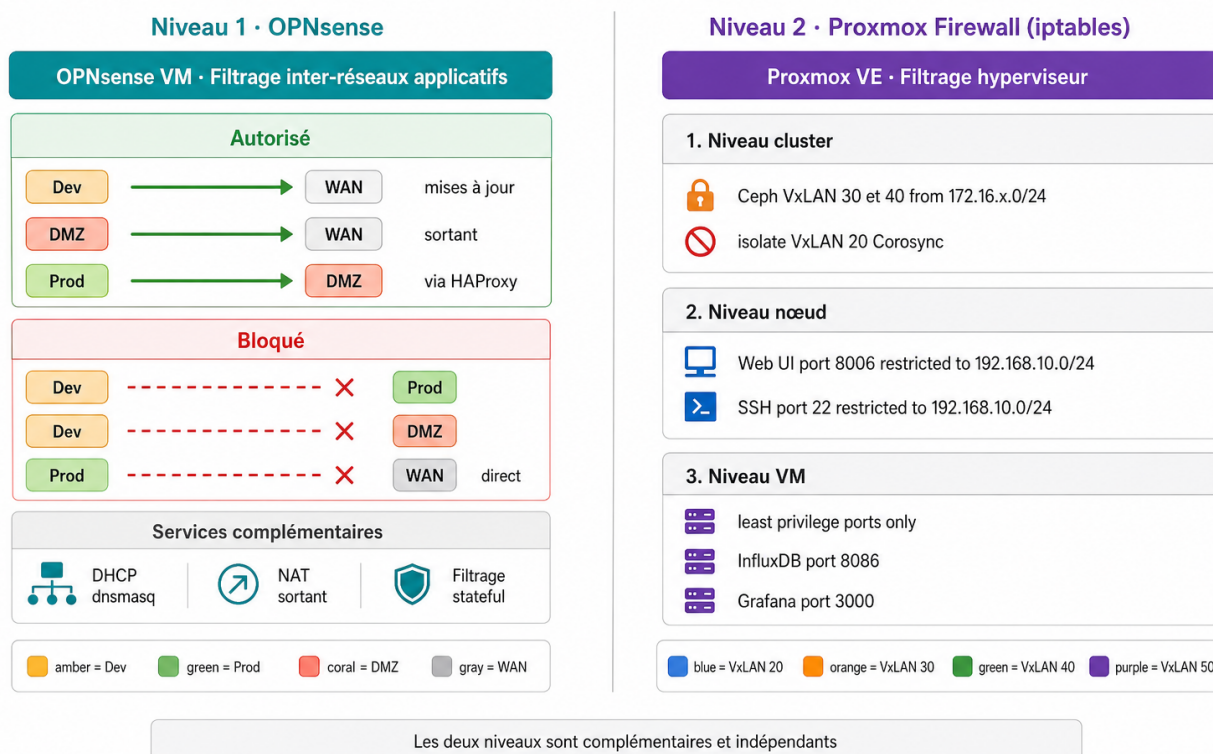
FIGURE III.8 – Architecture du Pare-feu : OPNsense et Proxmox Firewall
